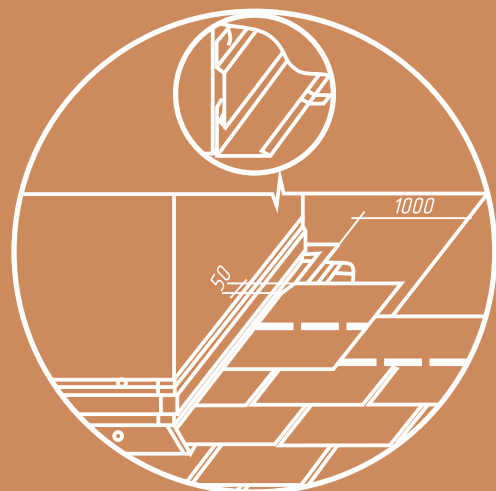
Вариант 1 Примыкание к стенам и трубам
